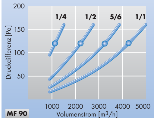
Anfangsdruckdifferenzkurven kennzeichnen den Haupteinsatzbereich ● Nennvolumenstrom
